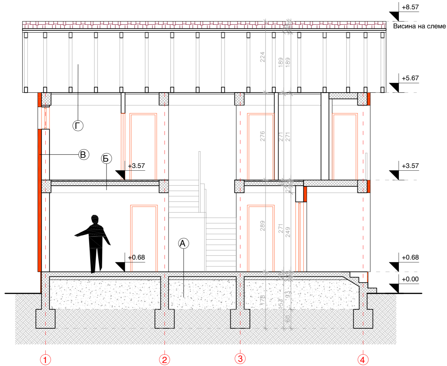
ПРЕСЕК 2-2
