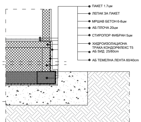
ДЕТАЛ 2
