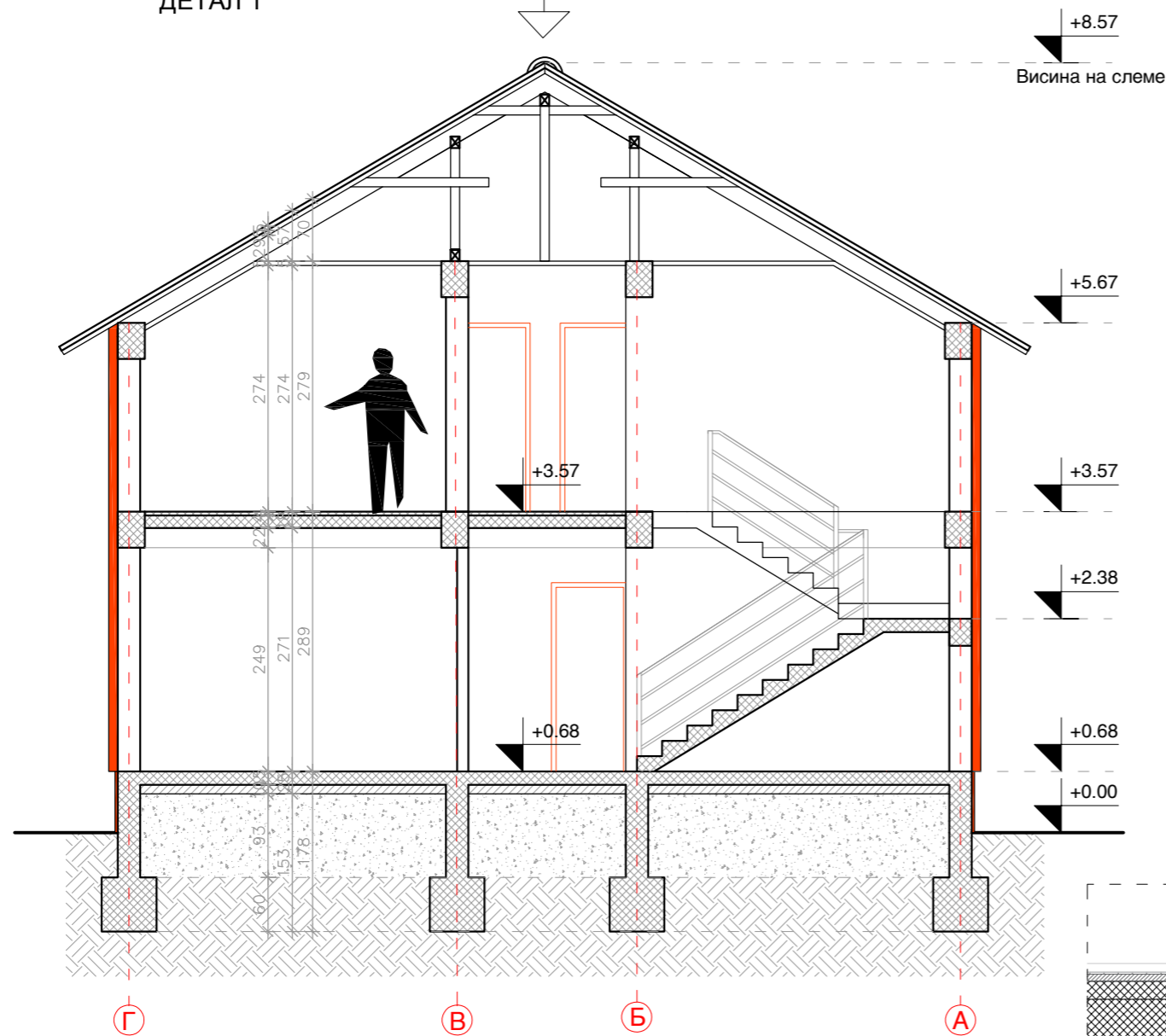
ПРЕСЕК 1-1
