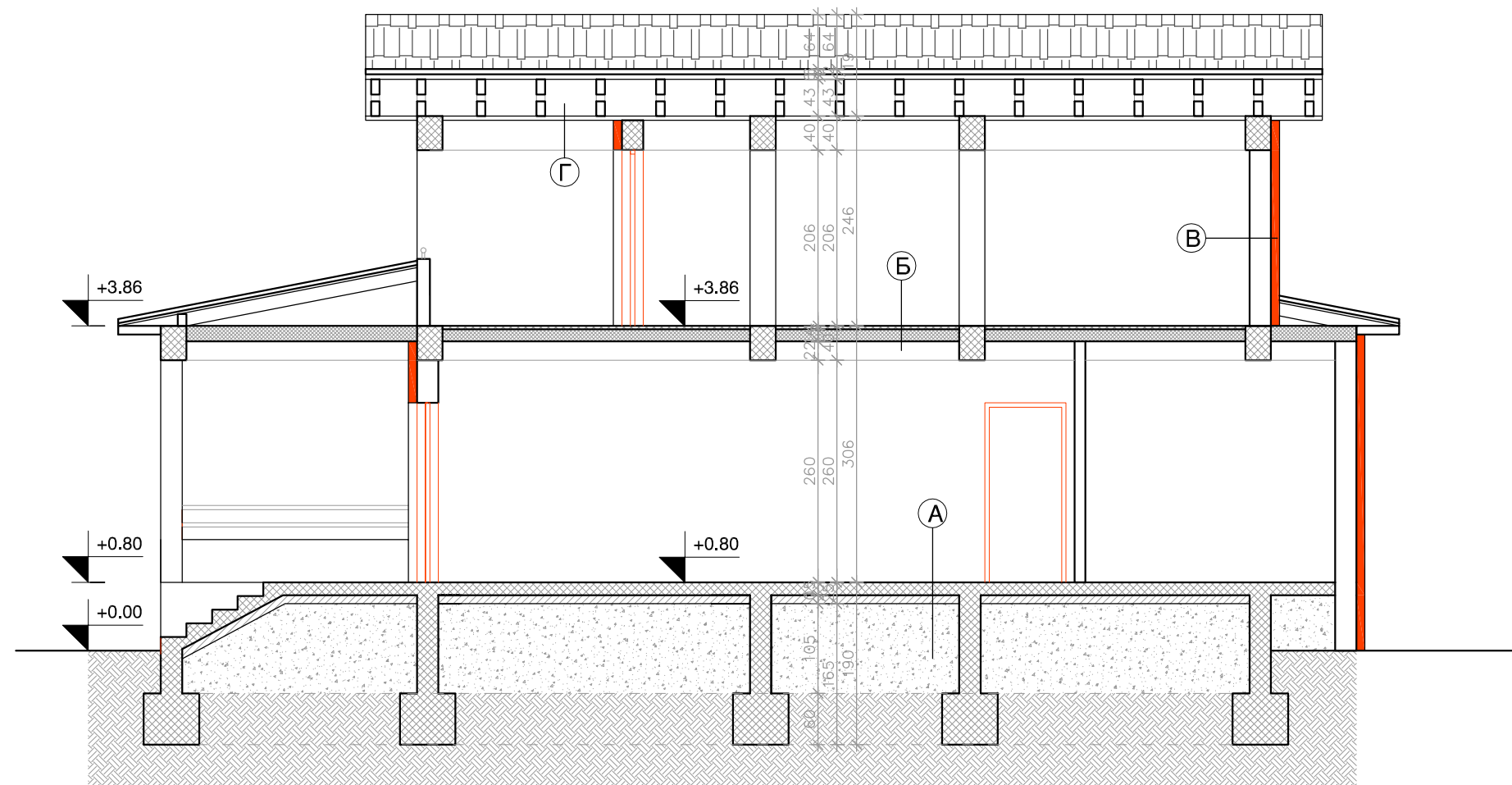
ПРЕСЕК 2-2
