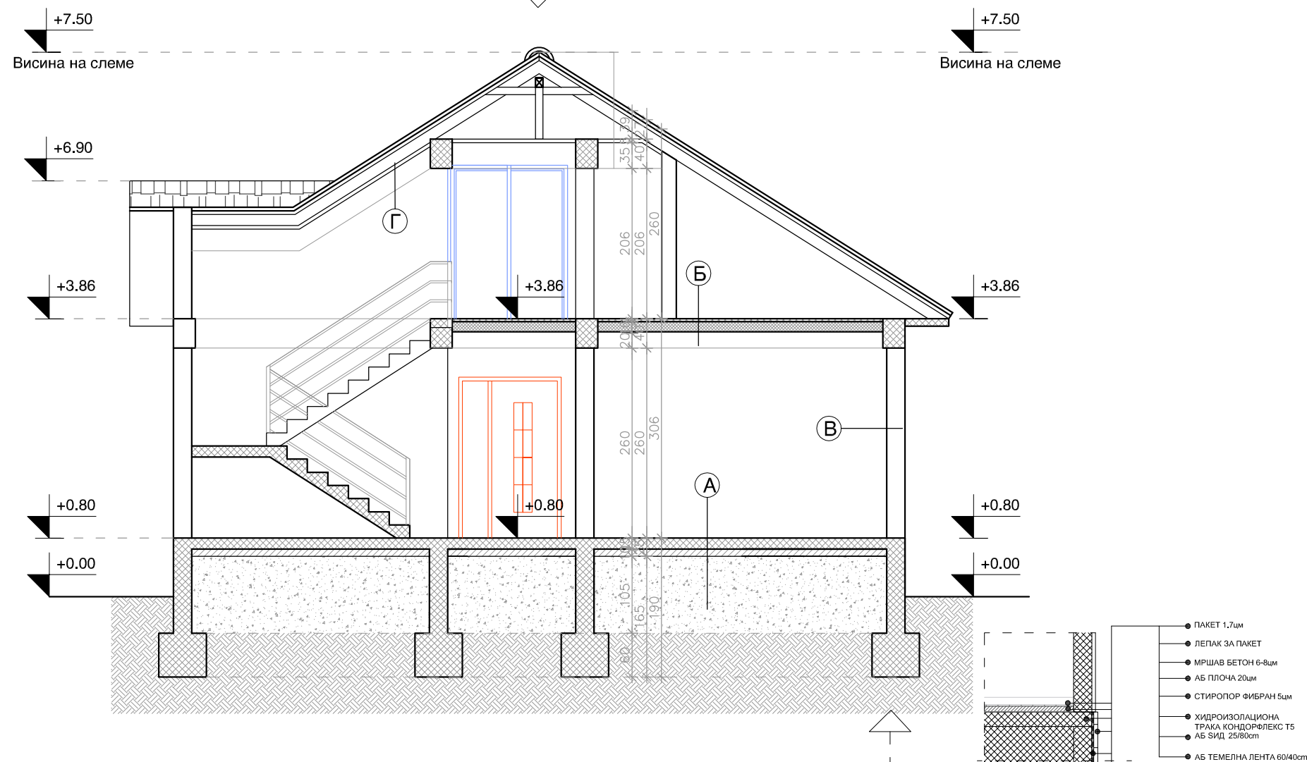
ПРЕСЕК 1-1
