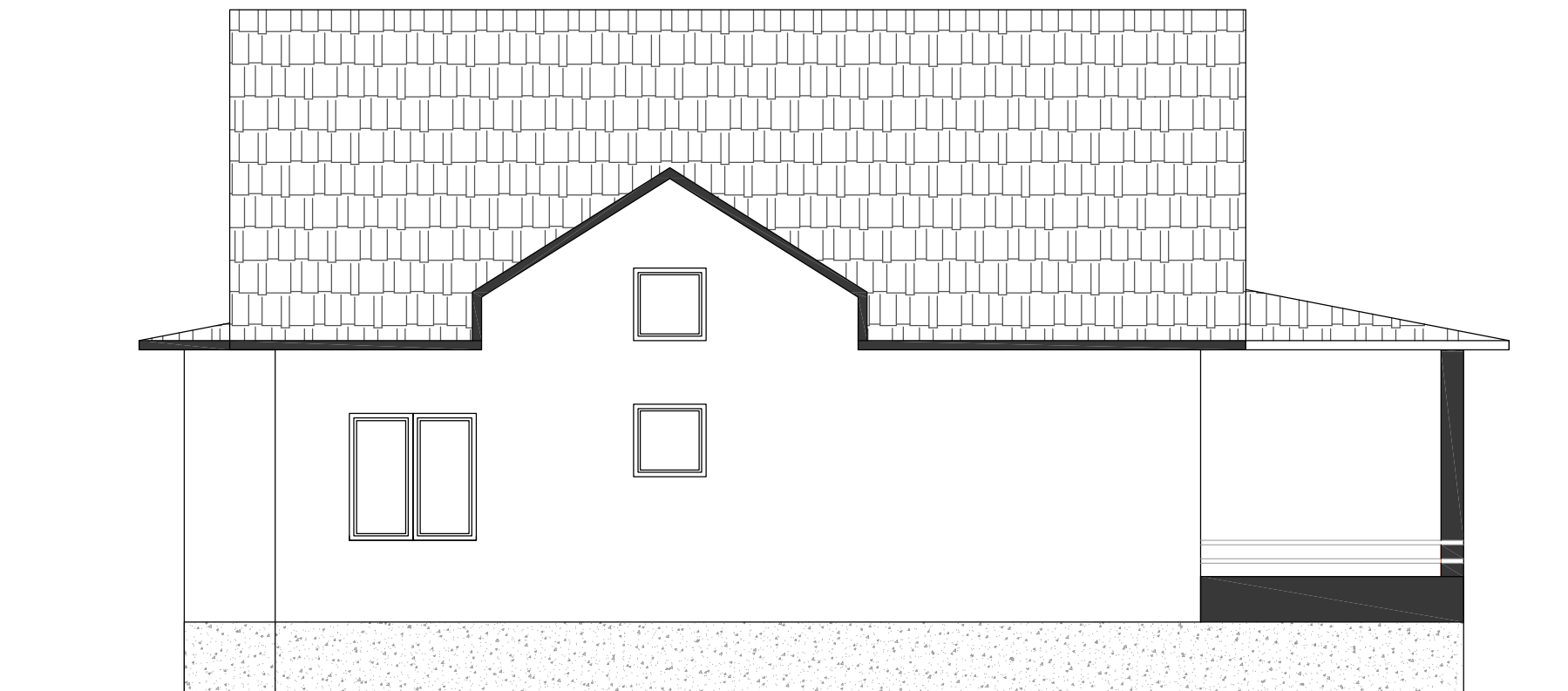
ЗАПАДНА ФАСАДА
