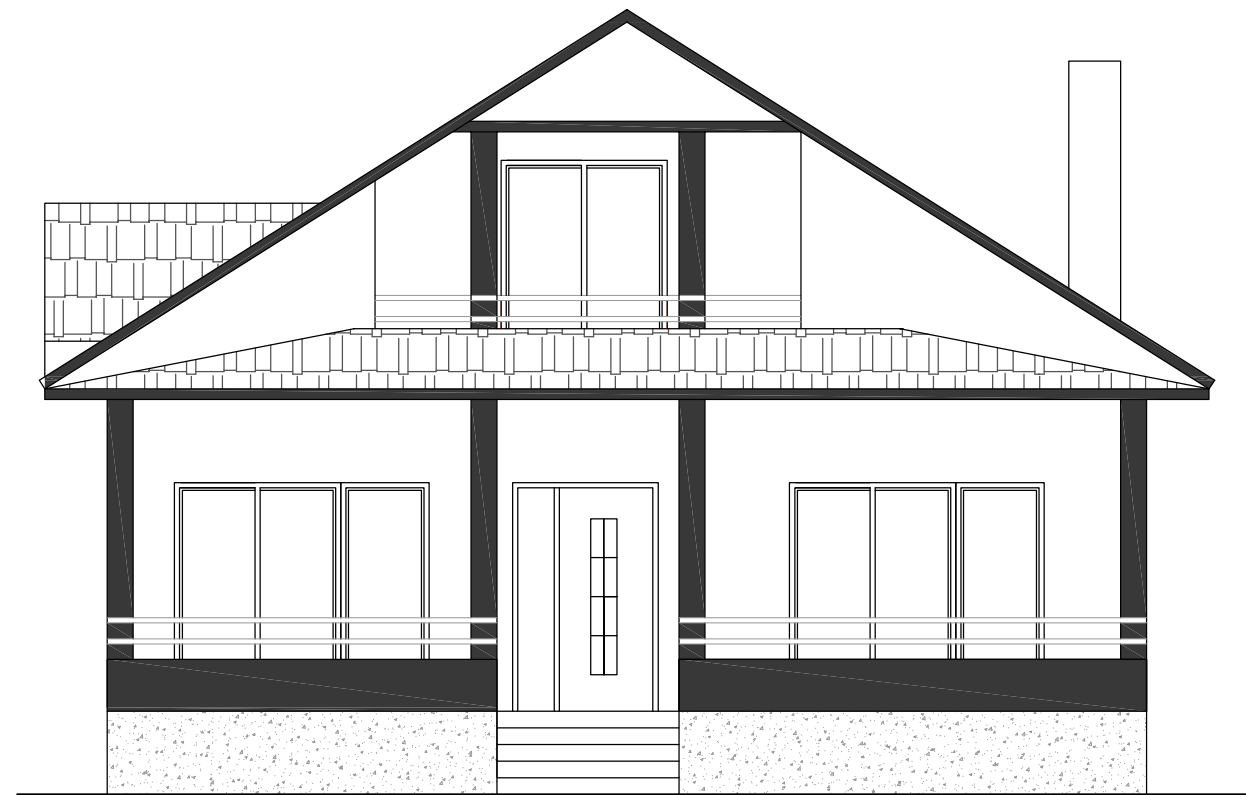
СЕВЕРНА ФАСАДА
