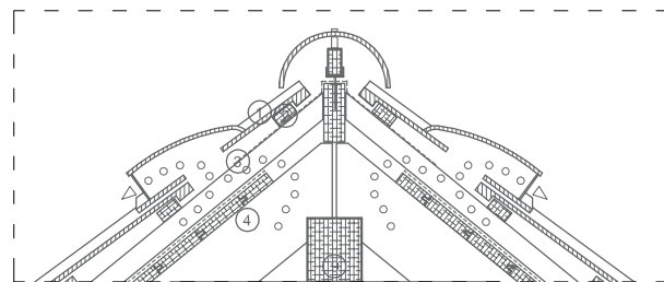
ДЕТАЛ 1
