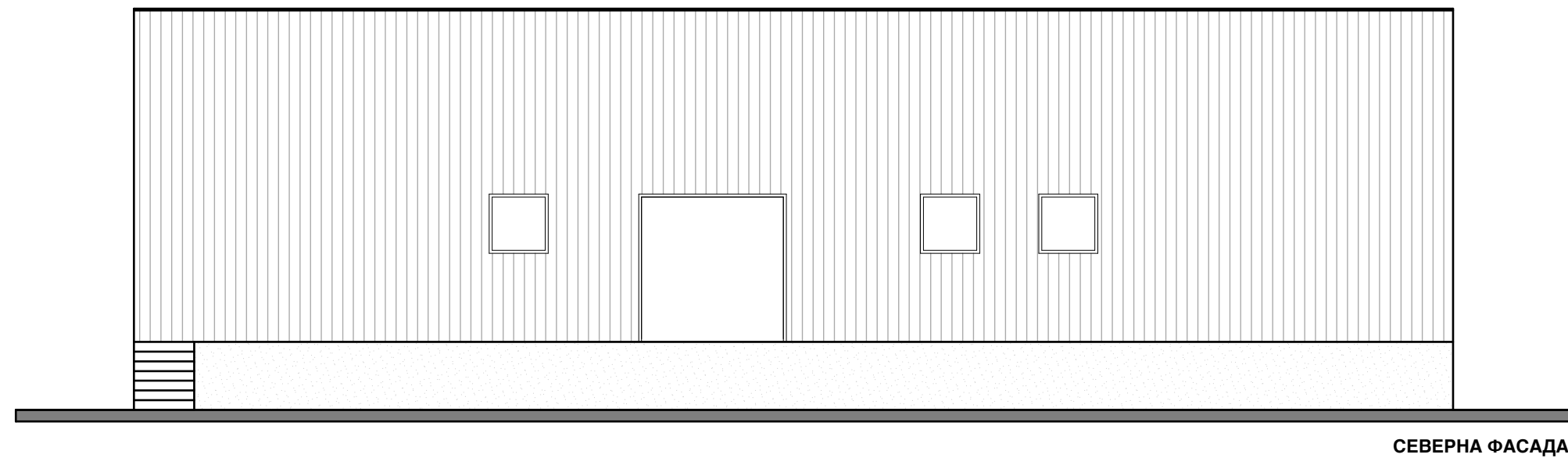
СЕВЕРНА ФАСАДА
