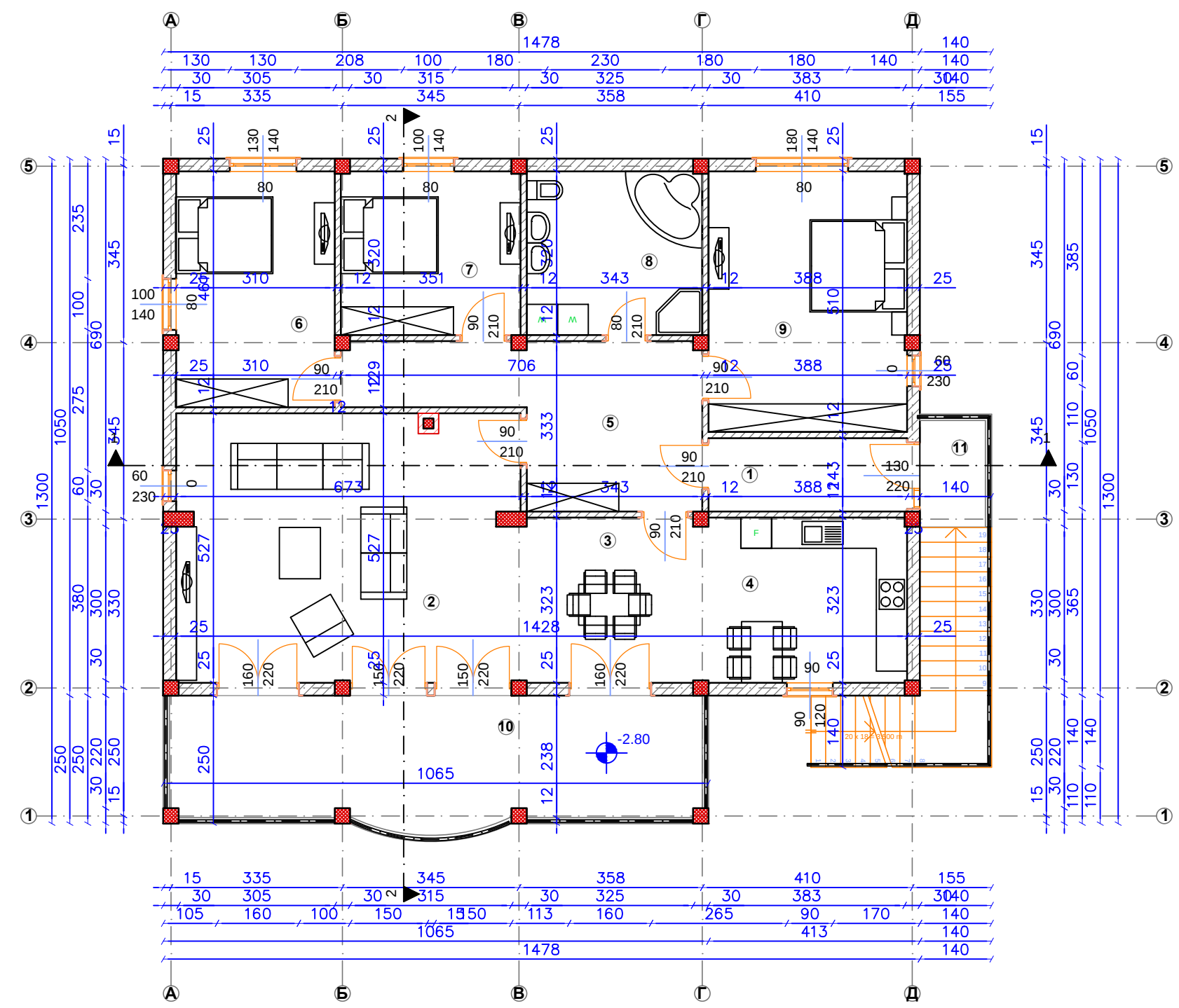
ОСНОВА НА ПРВИ КАТ, КОТА +2,80
