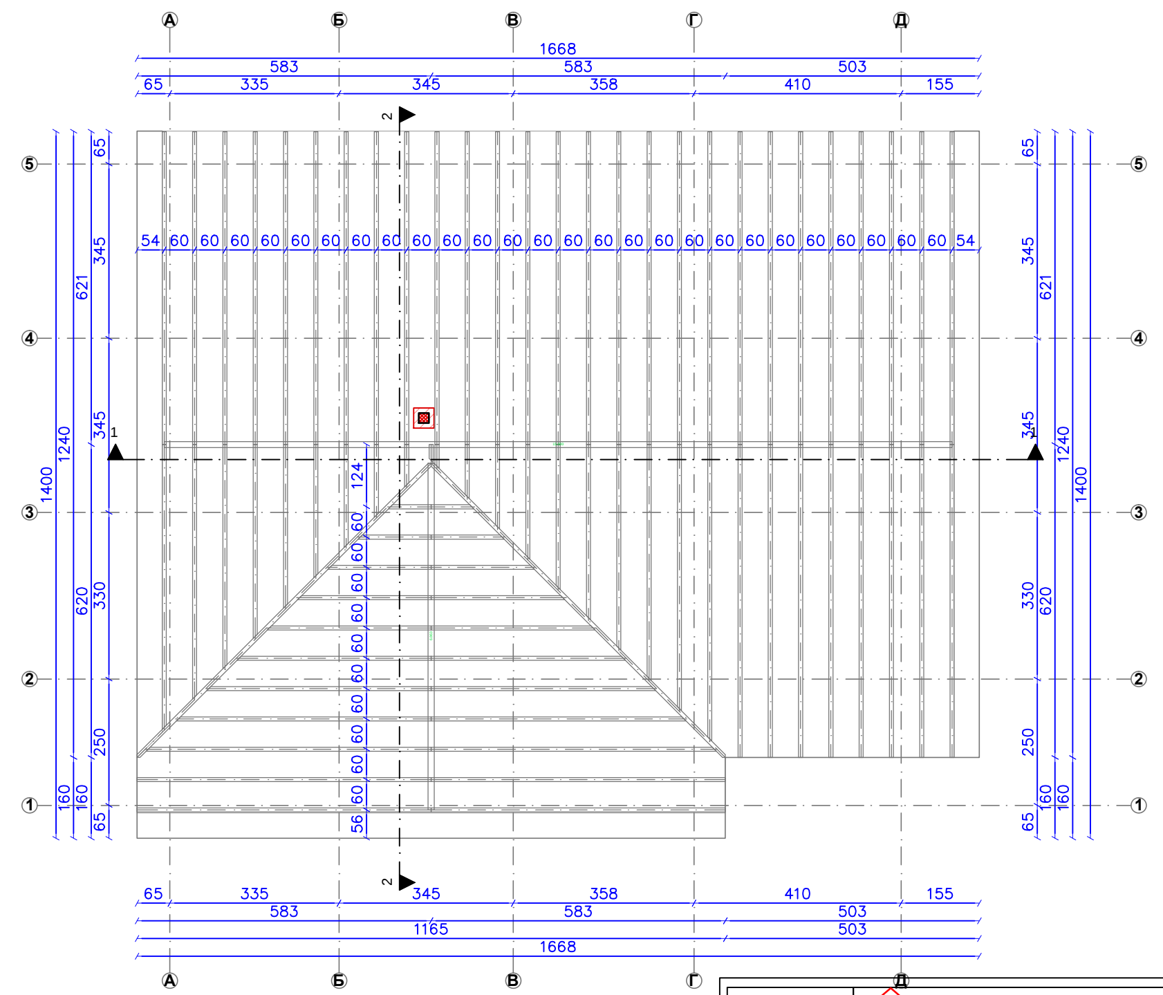
ОСНОВА НА КРОВНА КОНСТРУКЦИЈА, КОТА +9,08
