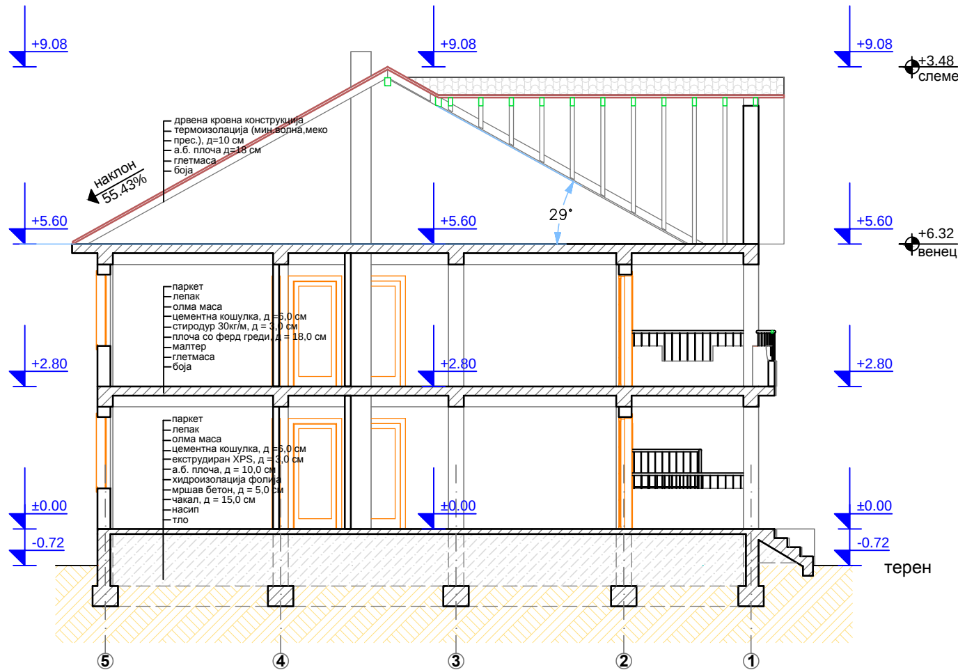
ПРЕСЕК 2-2
