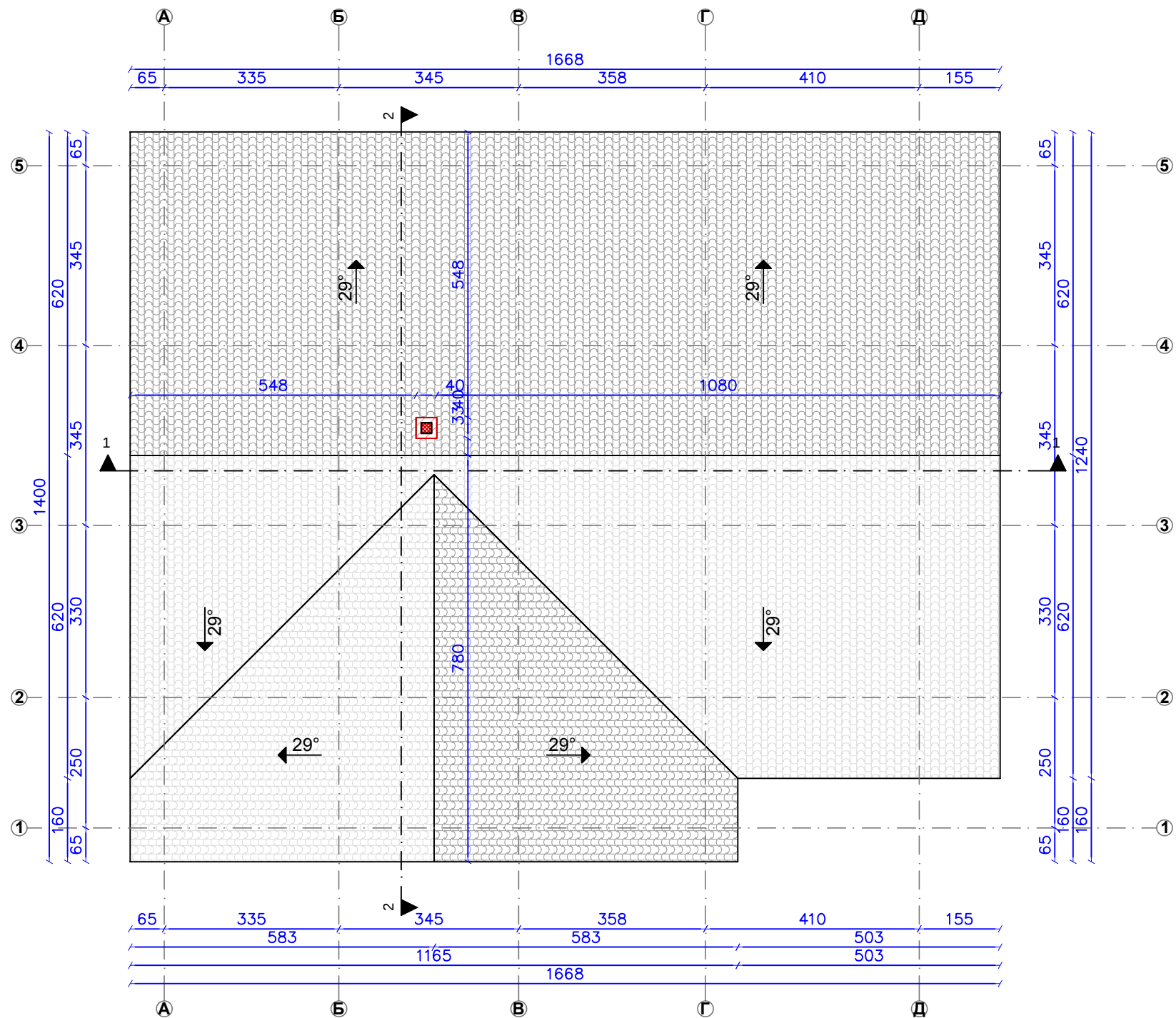
ПЕТТА ФАСАДА, КОТА +9,08
