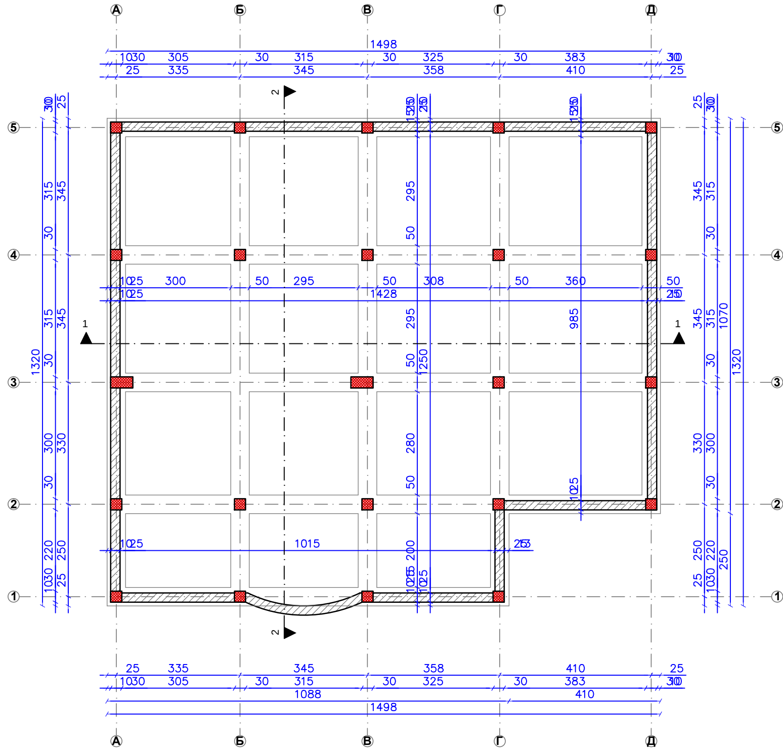
ОСНОВА НА ТЕМЕЛИ
