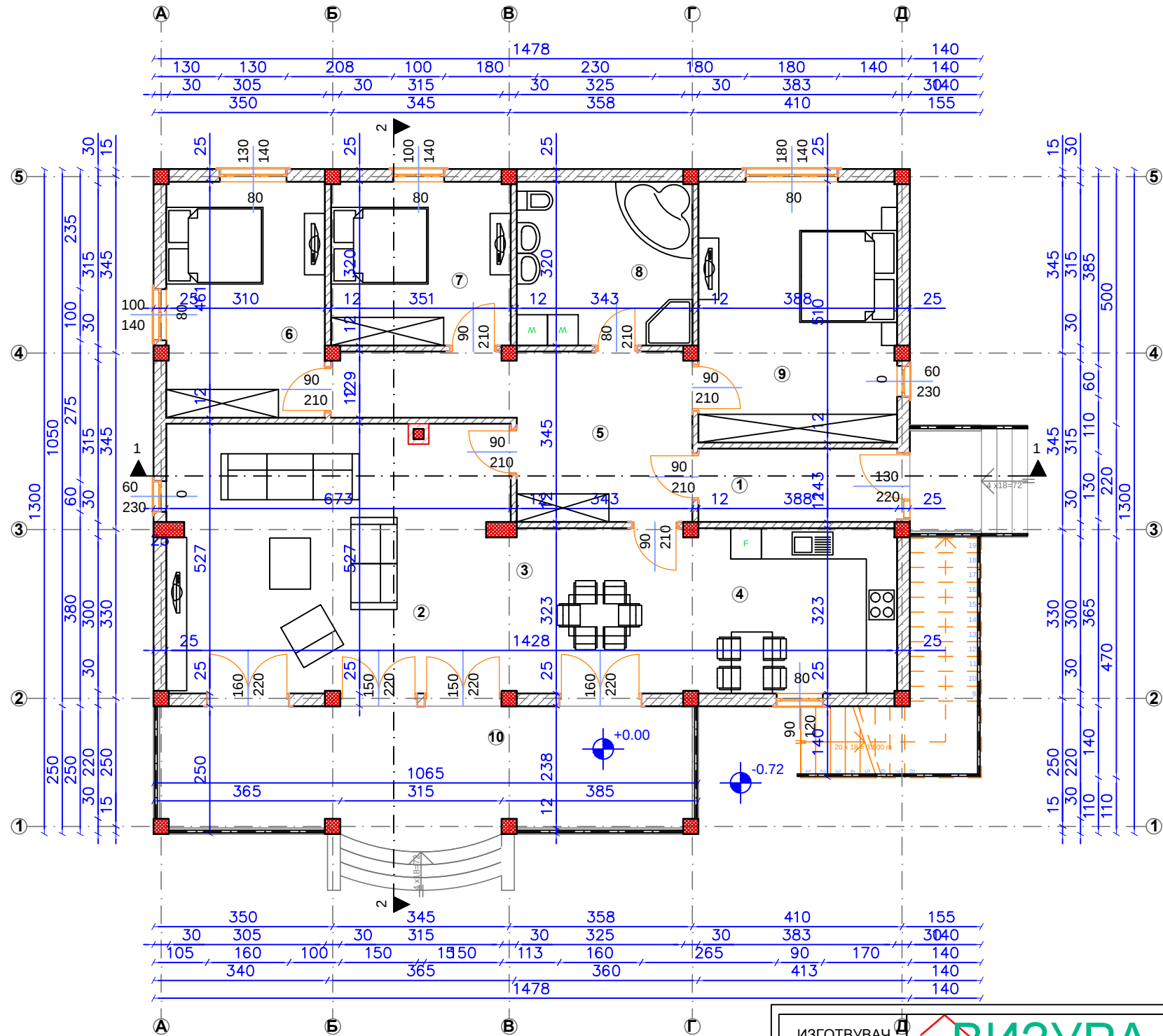
ОСНОВА НА ПРИЗЕМЈЕ, КОТА ±0,00
